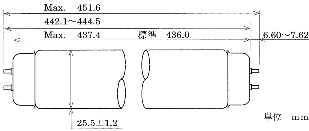
昼光色蛍光ランプ（直管形） 〈サンライン〉
